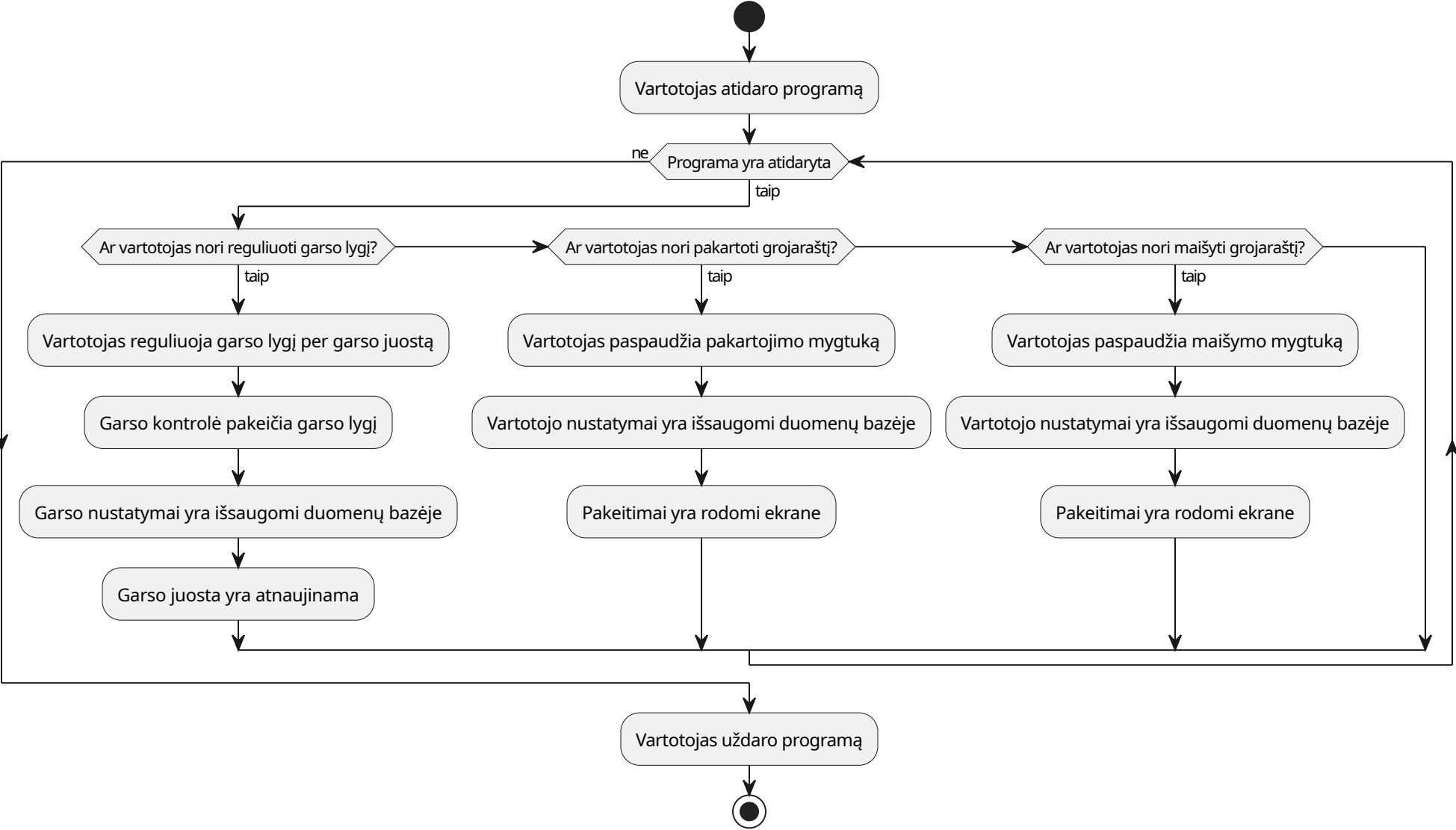
Vartotojo nustatymų valdymo diagrama
